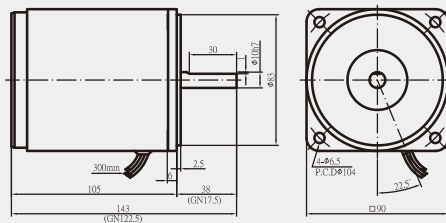
20W 5TK20A(GN)-AP(CP)
