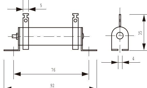
DDR20W20Ω J (20/20)
