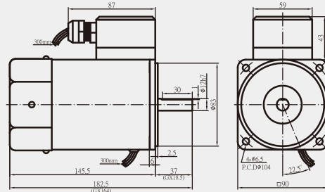
40W 5TK40CA(GN/GX)-AP(CP)
