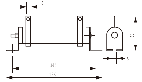
DDR80W50Ω J (80/50)
