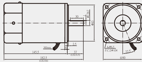
40W 5TK40A(GN/GX)-AP(CP)
