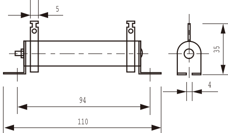
DDR30W20Ω J (30/20)
